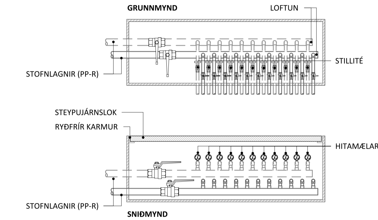
DEILIKISTA SNJÓBRÆDSLULA 1 : 20
