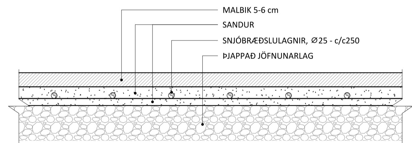
KENNISNIÐ SNJÓBRÆDSLULA MALBIK 1 : 10
