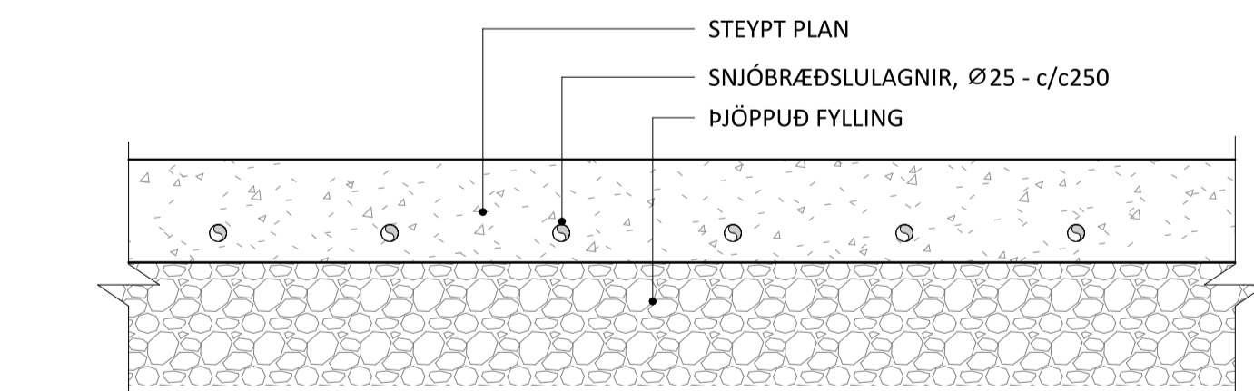
KENNISNIÐ SNJÓBRÆDSLULA STEYPA 1 : 10
