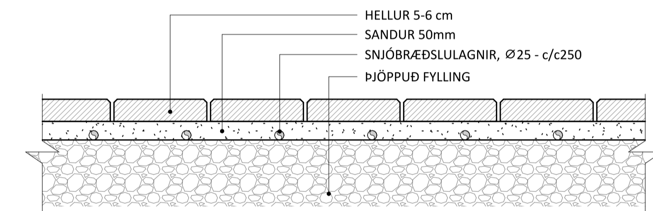
KENNISNIÐ SNJÓBRÆDSLULA HELLUR 1 : 10
